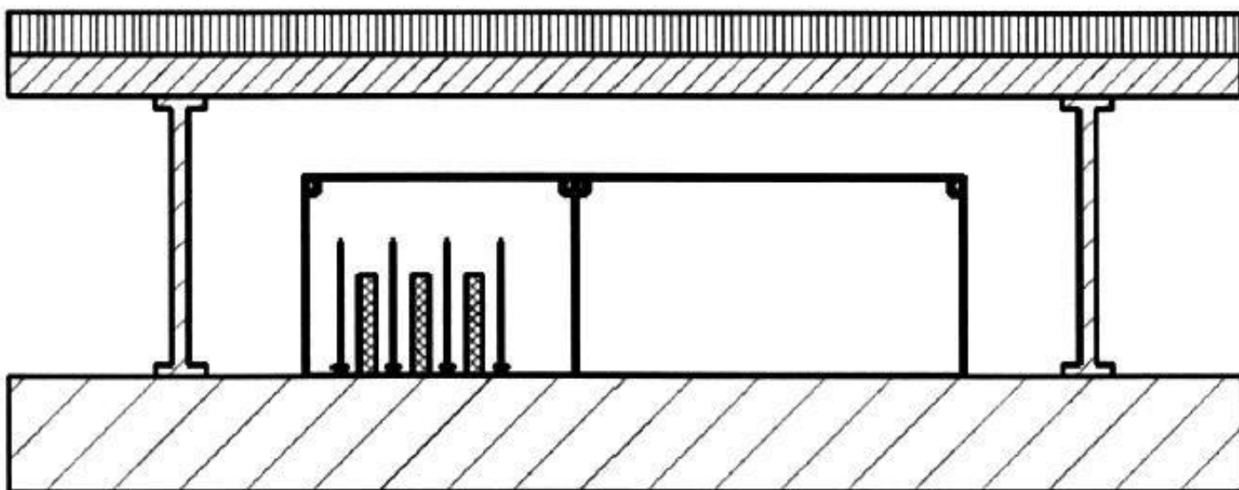
Рисунок АА.1б - Пример установки шинопровода в двойном полу Рисунок
