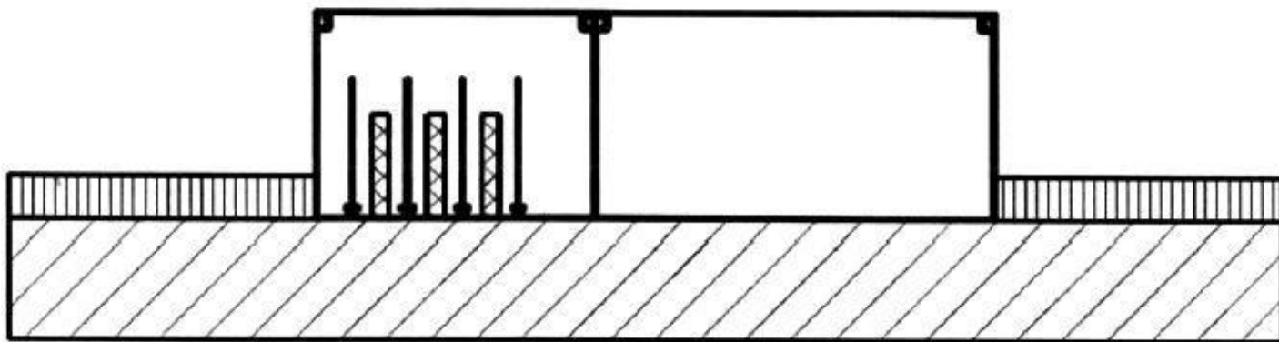
Рисунок АА.2 - Пример напольной установки шинопровода
