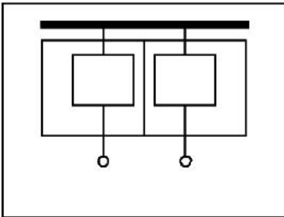
Вид 3а - Зажимы не отгорожены от шин
